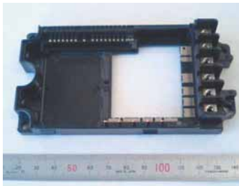
産業用端子台付モジュールケース industrial module cases with terminal blocks
